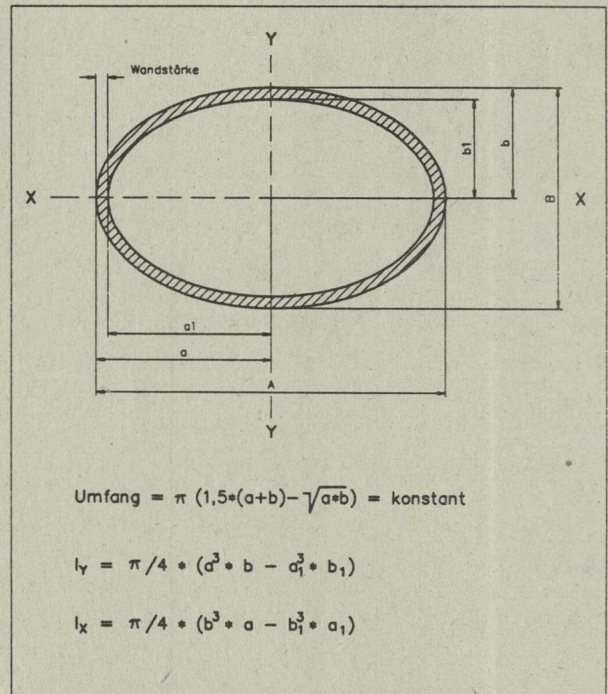
Bild 1. Grundlagen zur Berechnung der Querschnittskenngrößen von elliptischen Rohren
