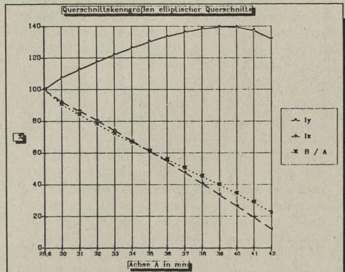
Bild 3. Widerstand gegen Biegung um die senkrechte Achse
