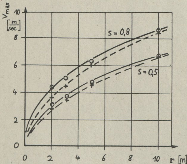
Bild 5: Abhängigkeit der maximalen Kurvengeschwindigkeit vom Kurvenradius und der Lage des Fahrzeugschwerpunktes Typ 1: —○— Typ 2: - - + - -
