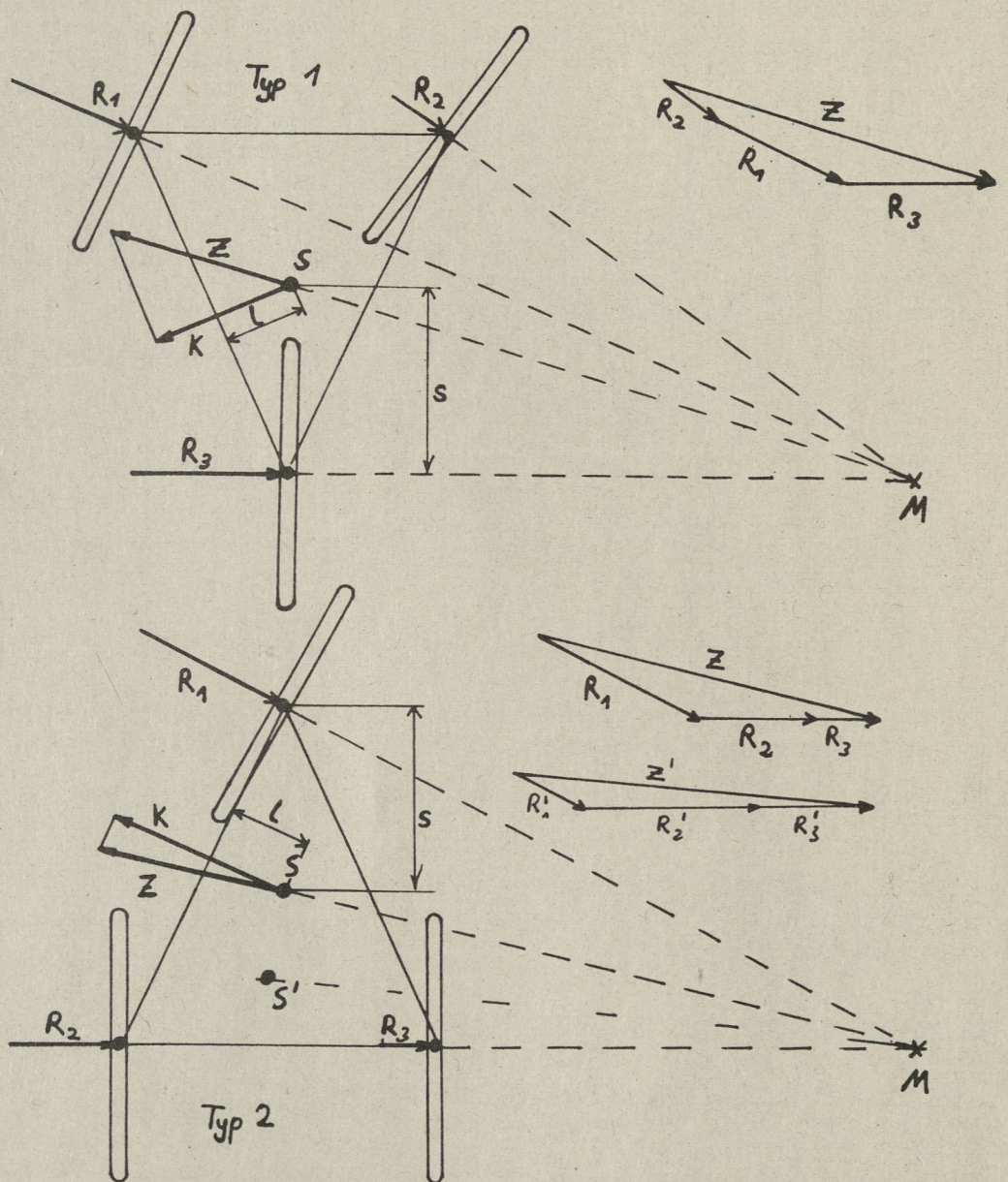
Bild 3: Kräfte am Dreirad beim Kurvenfahren
