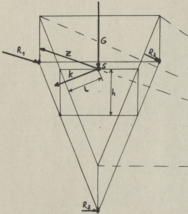
Bild 4: Räumliche Darstellung der Kräfte beim Kurvenfahren
