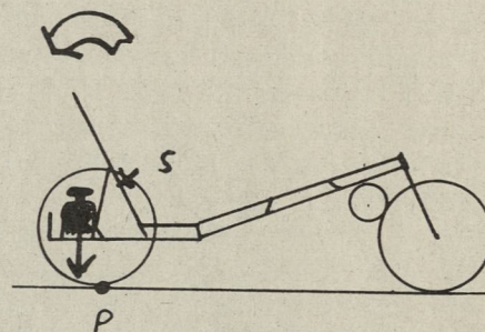
Bild 7: Ursachen für Überkippen oder zu geringe Haftung des Einzelrades Typ 1: Durch Bremsen der Vorderräder Typ 2: Durch Anfahrmoment oder hintere Last
