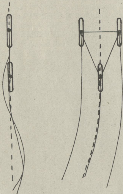
Bild 1: Lage der Radaufstandspunkte und Spur der Räder beim Zwei- und Dreirad
