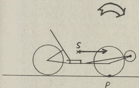
Bild 7: Ursachen für Überkippen oder zu geringe Haftung des Einzelrades Typ 1: Durch Bremsen der Vorderräder Typ 2: Durch Anfahrmoment oder hintere Last
