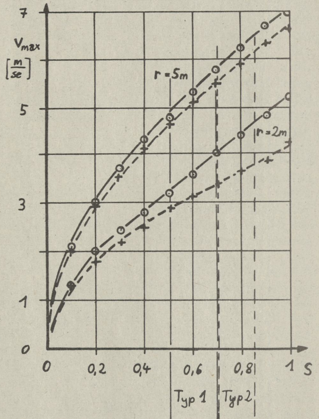
Bild 6: Abhängigkeit der maximalen Kurvengeschwindigkeit von der Schwerpunktlage - Darstellung für zwei verschiedene Kurvenradien Typ 1: —○— Typ 2: - - + - -
