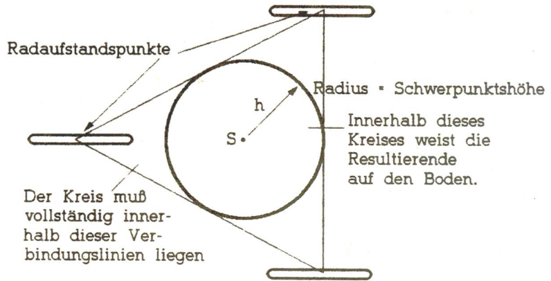
Bild 2: Konstruktion der Aufstandsfläche für ein kippsticheres Fahrzeug (Ansicht von oben)
