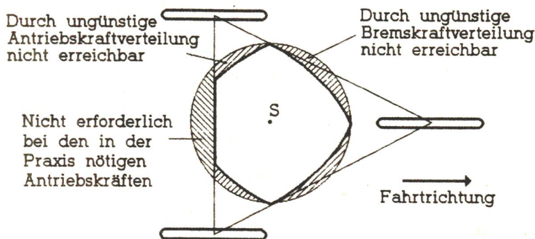
Bild 3: Verkleinerung der Aufstandsfläche durch Einschränkungen aus der Praxis (Ansicht von oben)
