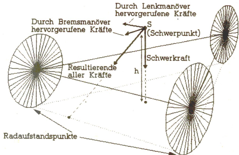
Bild 1: Schwerpunktlage und angreifende Kräfte (perspektivisch)
