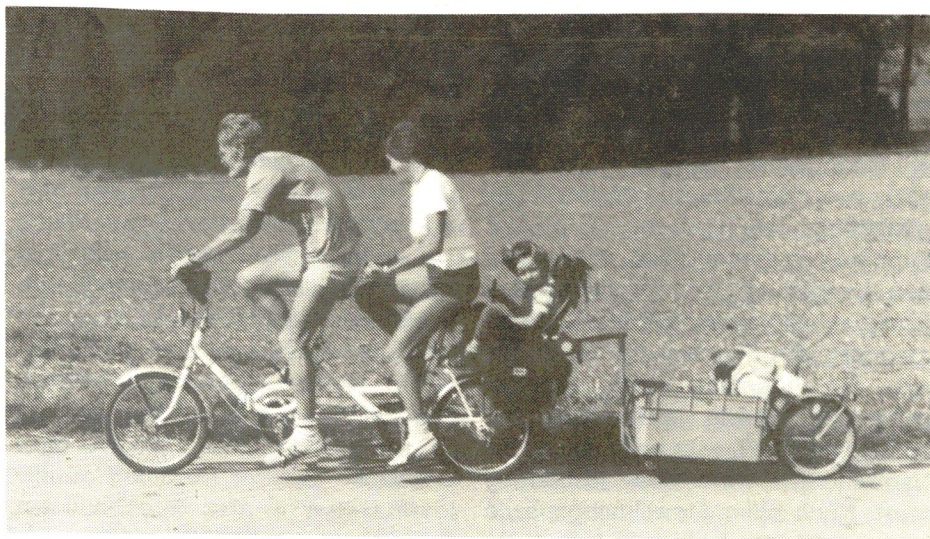
Gespann mit WIPO Fahrradanhänger "Radelboy". Die umgebaute Deichsel nebst Kupplung ermöglicht es, den Gepäckträger des Zugfahrzeugs voll zu nutzen, hier sogar mit einem Kindersitz.
