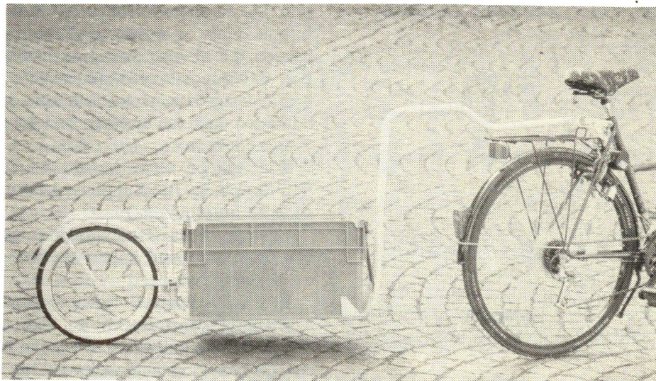
WIPO Fahrradanhänger "Radelboy" mit langer Deichsel und modifizierter Kupplung an der Sattelschranbe
