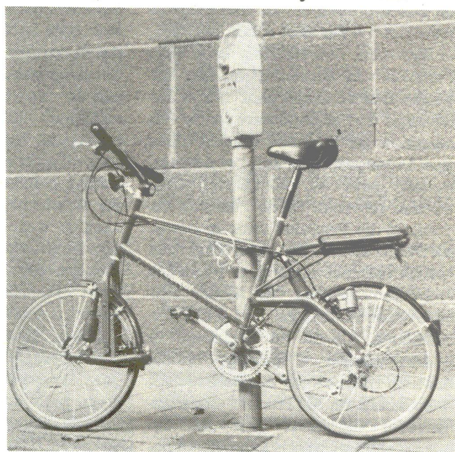
RADICAL - Stadtrad mit hydraulisch gedämpften Federungen aus den Niederlanden
