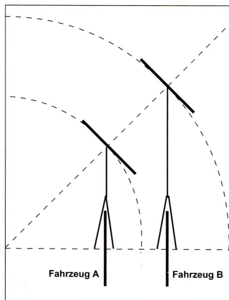
Bild 6: Kompaktlieger „Senkels easy“ ist trotz des größeren Radstandes um ca. 5 cm kürzer als die „Street Machine“. Erreicht wird dies durch die kleineren Laufräder (hintere 20“, vorne 16“) und die etwas aufrechtere Sitzposition.
