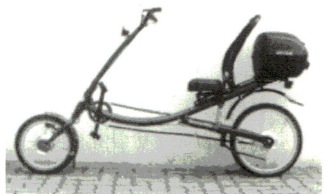
Bild 8: Langlieger „ScooterBike“ mit direkter Lenkung
