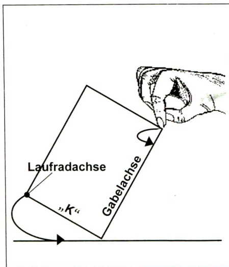
Bild 10: Simulation der Rahmenanhebung bei kräftigem Lenkereinschlag
