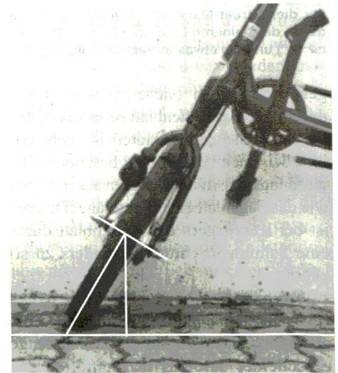
Bild 12: Rahmenabsenkung beim Lenkeinschlag. Beim Geradeauslauf hat die Nabe den Radius als Distanz zur Lauffläche (siehe Bild 9), beim Lenkeinschlag ist die Distanz kürzer.
