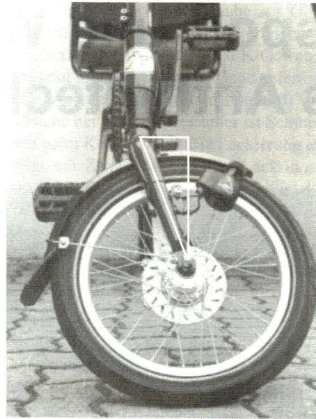
Bild 13: Rahmenabsenkung beim Lenkeinschlag von vorne betrachtet.
