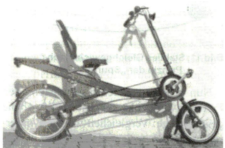
Bild 6: Kompaktlieger „Senkels easy“ ist trotz des größeren Radstandes um ca. 5 cm kürzer als die „Street Machine“. Erreicht wird dies durch die kleineren Laufräder (hintere 20“, vorne 16“) und die etwas aufrechtere Sitzposition.
