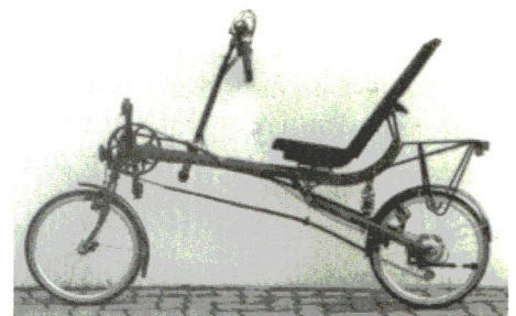
Bild 7: Kompaktlieger „Red Pepper“ mit indirekter Lenkung oben
