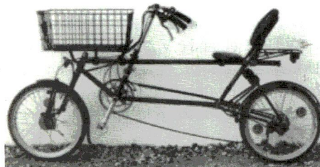
Bild 1: Langlieger „atl“ mit 20“-Laufrädern vorne und hinten
