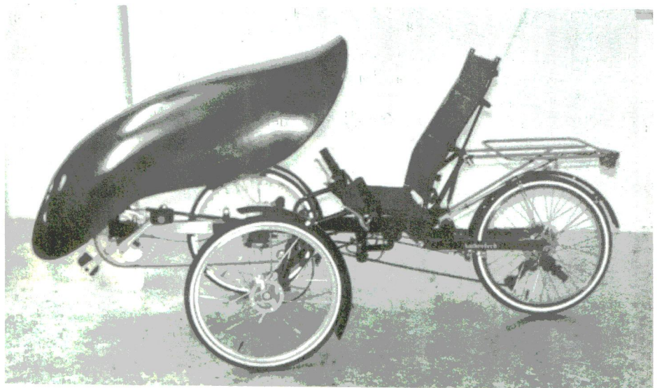
Anthrotech-Trike mit Räderwerk-Frontverkleidung
