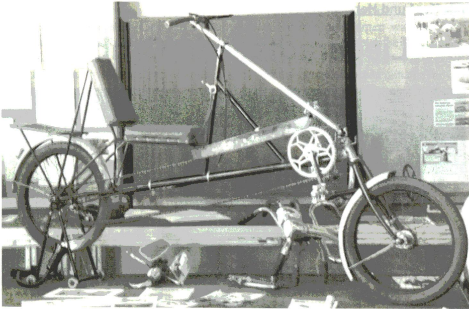
Restauriertes Mochet-Liegerad aus den 30er Jahren
