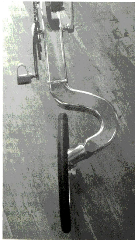
Liegerad DIMA aus Alu-Blech geformte Profil-Bauweise mit Achsschenkelenkung vorne (siehe zu diesem Fahrzeug ausführliches Typenblatt in PRO VELO 26, S. 40)
