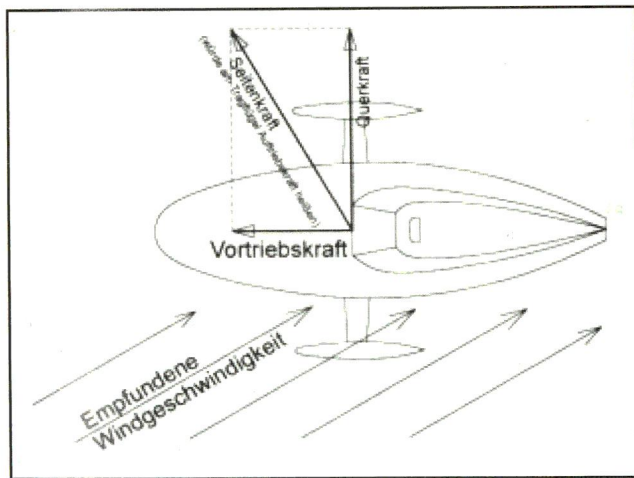
Bild 11: Die durch Seitenwind hervorgefufenen Kräfte am aerodynamisch günstig gestalteten Velomobil
