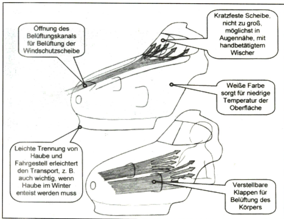
Bild 2: Beispiel für Hauptteil einer Velomobilverkleidung
